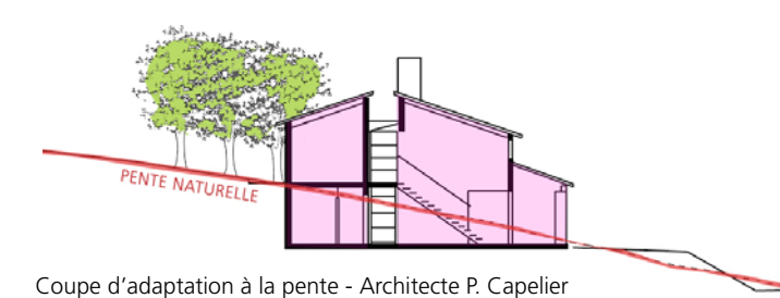
Coupe d'adaptation à la pente - Architecte P. Capelier
