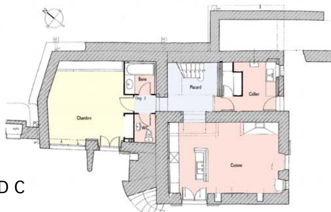
Etage
