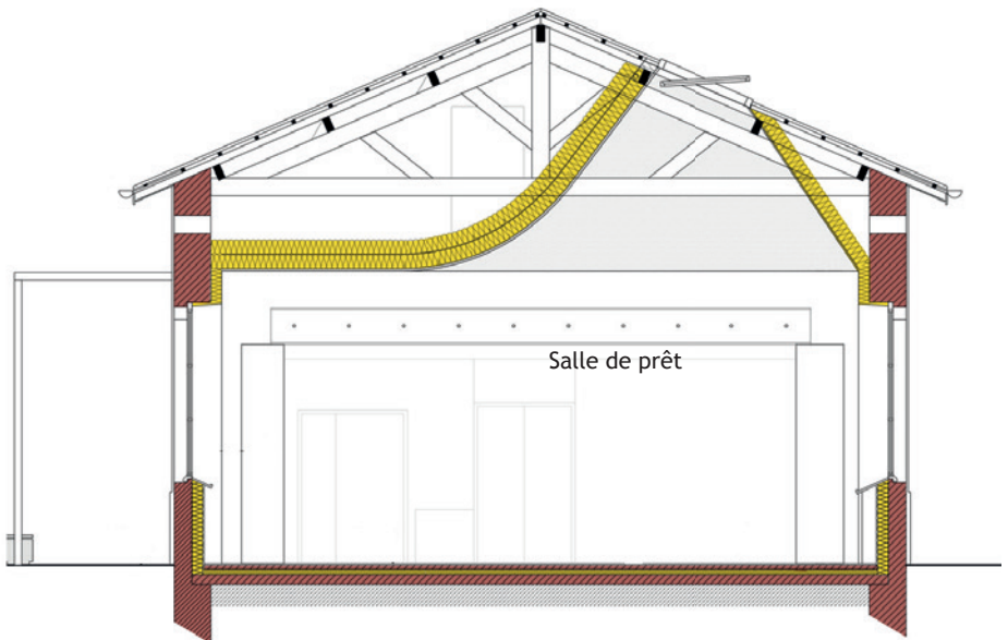
Coupe sur le puits de jour, au Nord
