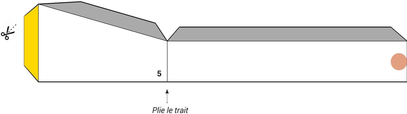
Murs appentis de la borde lauragaise - PATRON 5
