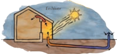
Association d'un puits géothermique et d'une serre
